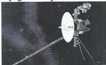
Voyager 1
